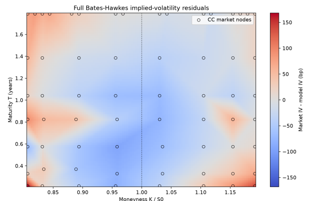
(d) Full Bates–Hawkes
